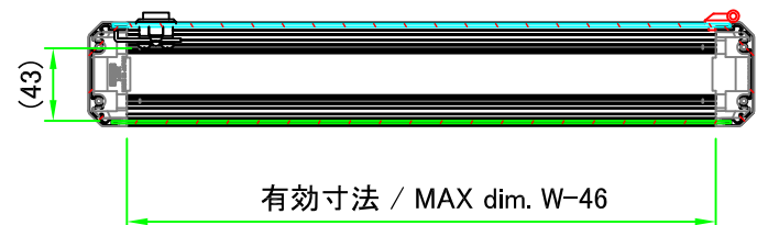
A-A (1:5)
